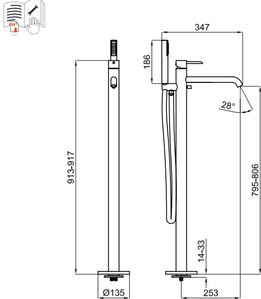
Техническая схема
